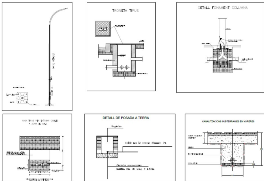
Detalls constructius
